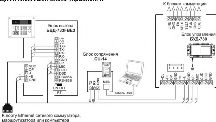
Рисунок 17.1 - Схема соединений блока вызова с блоком управления БУД-730 и блоком сопряжения СУ-14
