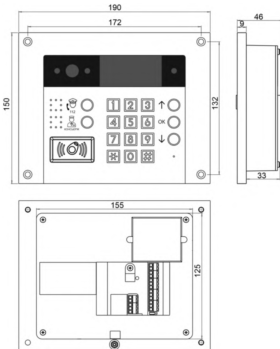
Рисунок 7.2 – Установочные размеры блока вызова
