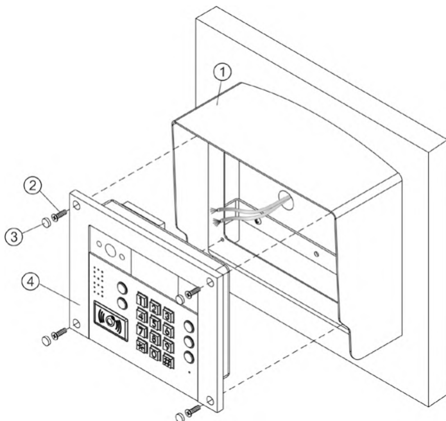
Рисунок 7.5 - Установка блока на монтажный комплект MKF-432
