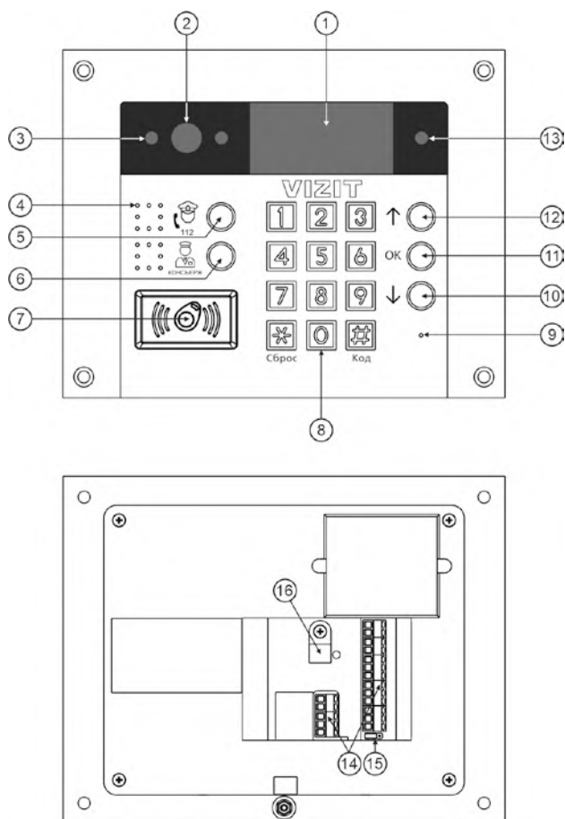
Рисунок 2.1 - Внешний вид блока вызова
