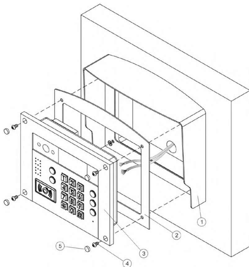
Рисунок 7.4 - Установка блока вызова на монтажный комплект МК-432
