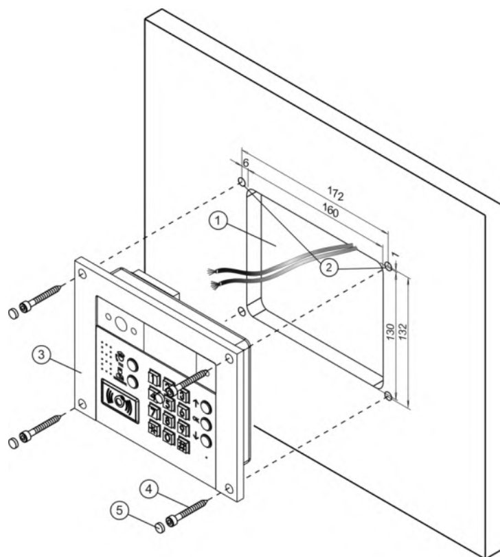
Рисунок 7.3 - Крепление блока вызова на неподвижную часть металлической двери
