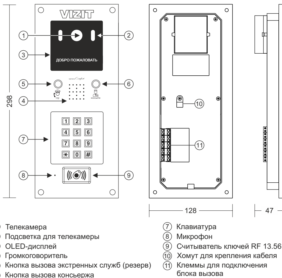
Рисунок 1 - Внешний вид и органы управления блока
