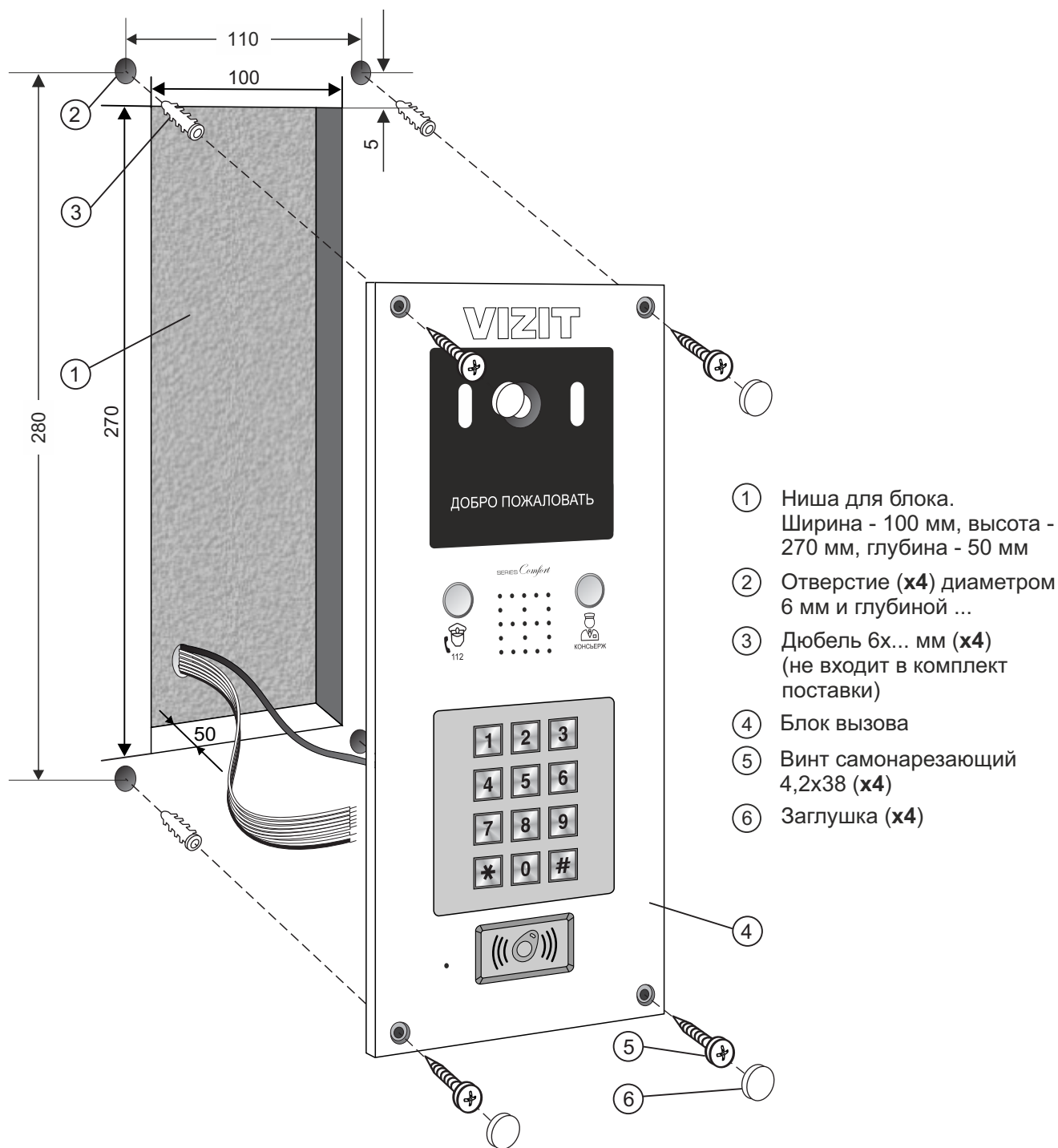
Рисунок 2 - Установка блока на стену
