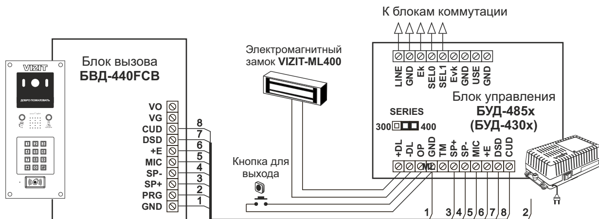
Рисунок 6 - Схема соединений блока вызова БВД-440FCB с блоком управления БУД-485х (БУД-430х) , электромагнитным замком VIZIT-ML400 и кнопкой для выхода
