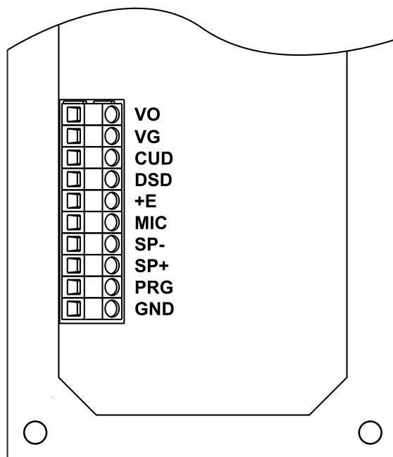
Рисунок 4 - Расположение клемм
