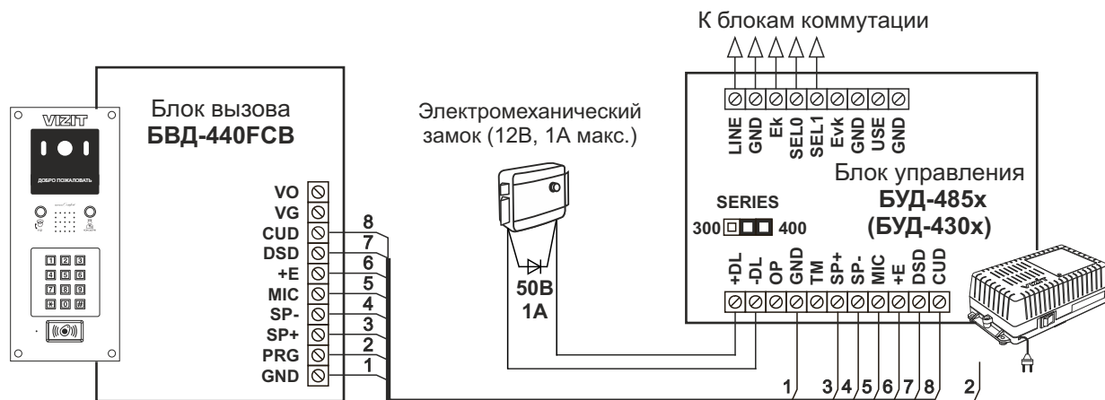
Рисунок 7 - Схема соединений блока вызова БВД-440FCB с блоком управления БУД-485х (БУД-430х) и электромеханическим замком
