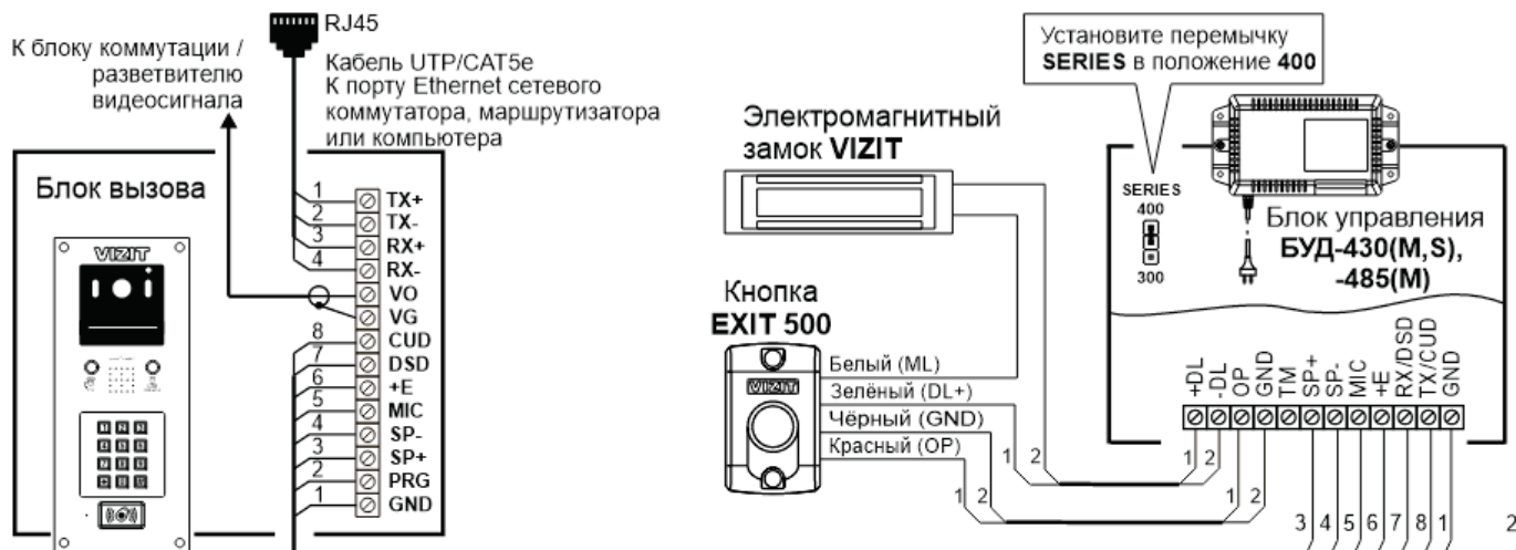
Рисунок 8.1 – Схема соединений блока вызова с блоком управления БУД-430(М,С), -480(С), -485(М), электромагнитным замком VIZIT-ML400 и кнопкой EXIT 1000
