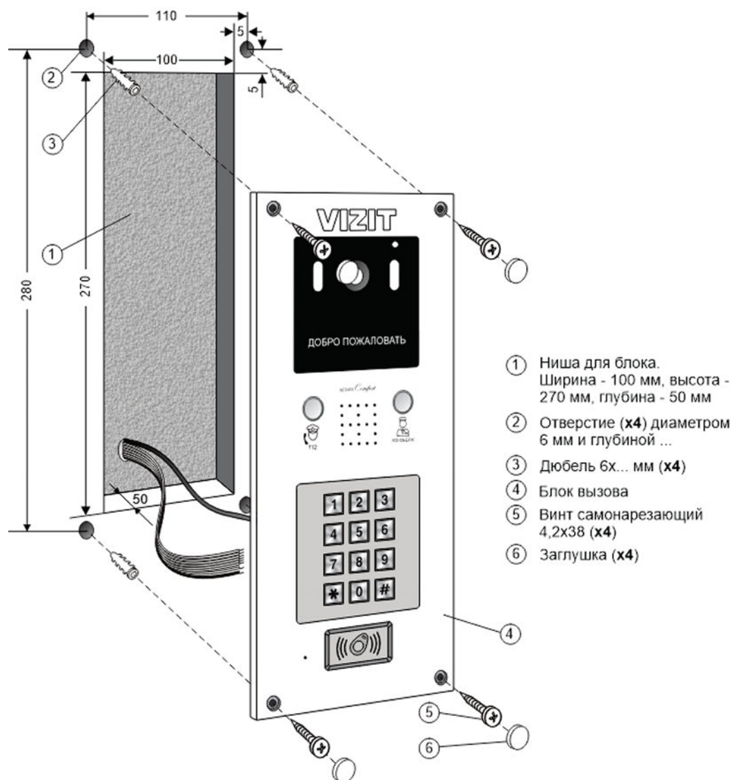
Рисунок 6.2 - Установка блока вызова на стену
