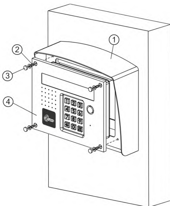
Рисунок 6.4 - Установка блока на монтажный комплект МКФ-432
