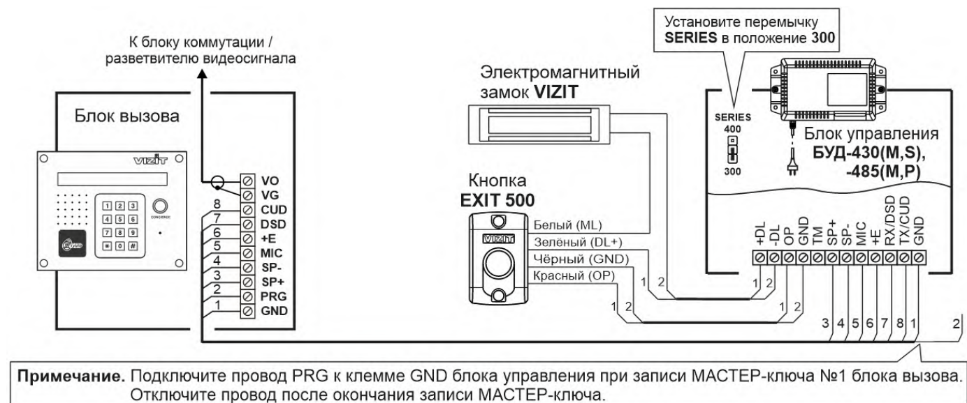
Рисунок 8.2 – Схема соединений блока вызова с блоком управления БУД-430(М,С), -485(М,Р), электромагнитным замком VIZIT-ML400 и кнопкой EXIT 500
