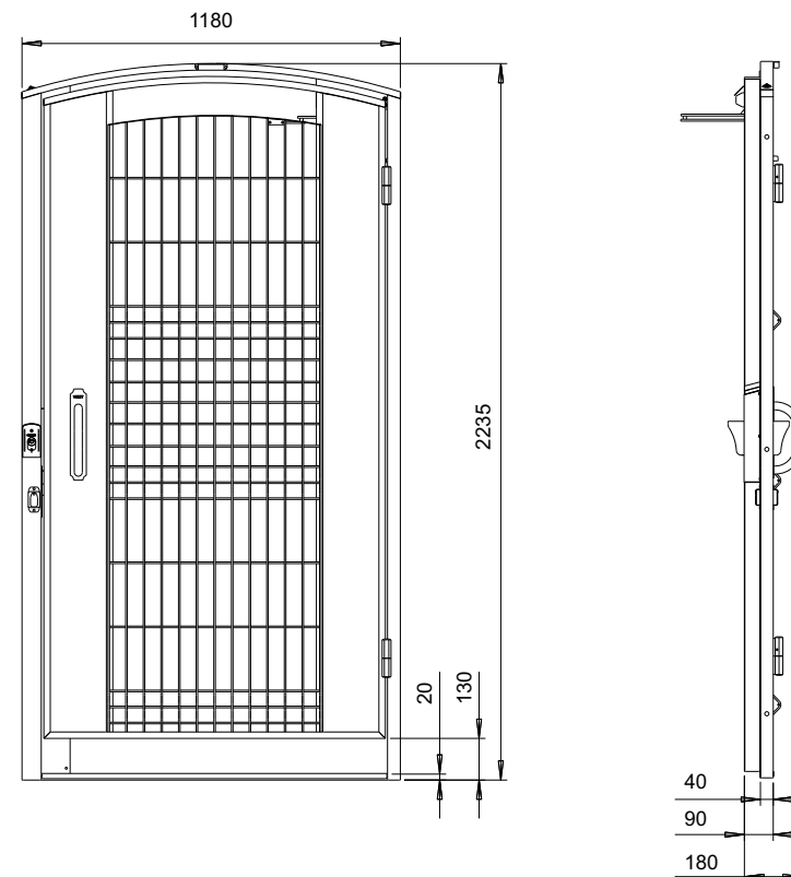
Рис. 2 - Габаритные размеры KCH-12
