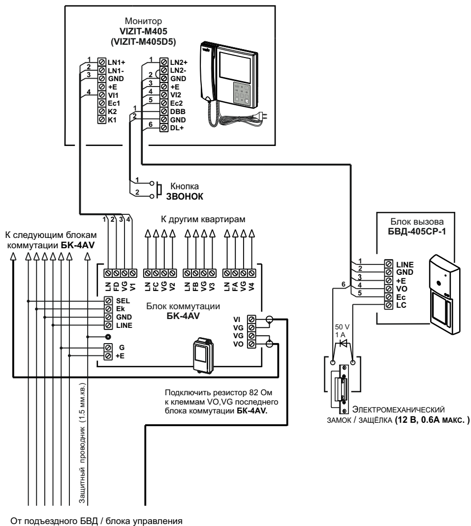
Рисунок 7 - Схема соединений монитора VIZIT-M405 (VIZIT-M405D5) с блоком коммутации БК-4AV , малоабонентским блоком вызова и кнопкой ЗВОНОК
