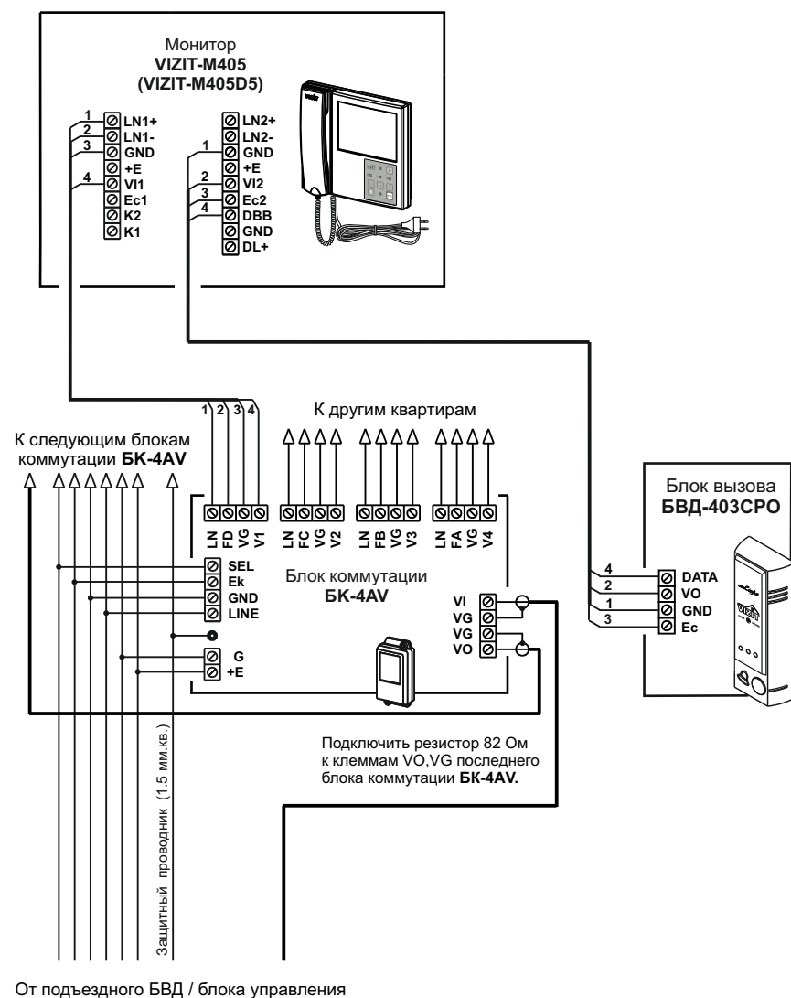
Рисунок 11 - Схема соединений монитора VIZIT-M405 (VIZIT-M405D5) с блоком коммутации БК-4AV и блоком вызова БВД-403CPO (телекамера + кнопка ЗВОНОК )
