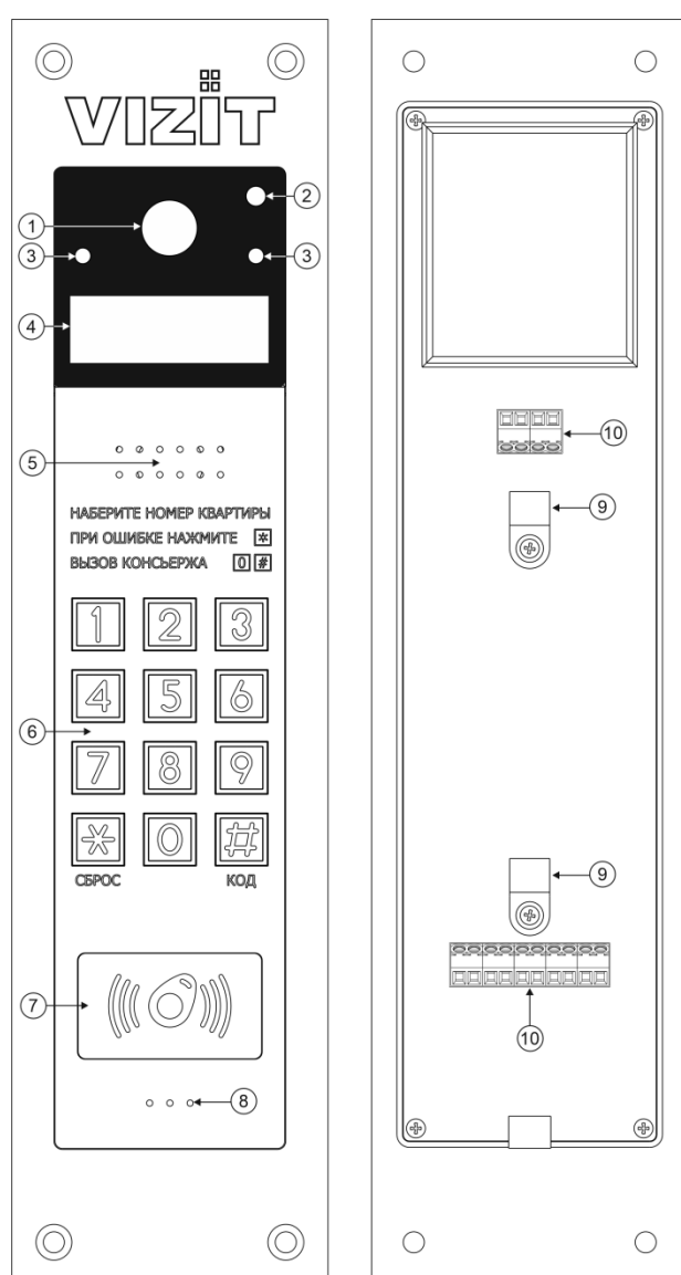
Рисунок 2.1 - Внешний вид блока вызова
