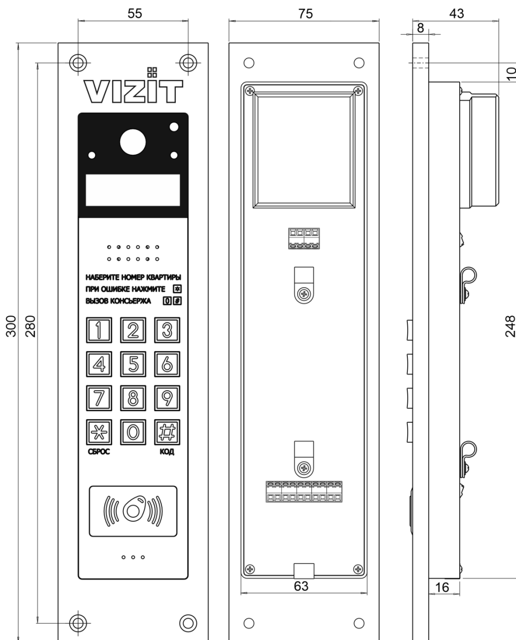
Рисунок 6.2 – Установочные размеры блока вызова
