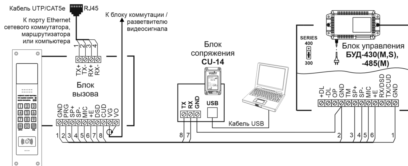
Рисунок 16.1 - Схема соединений блока вызова с блоками управления БУД-430(S, М), -485(М) и блоком сопряжения CU-14
