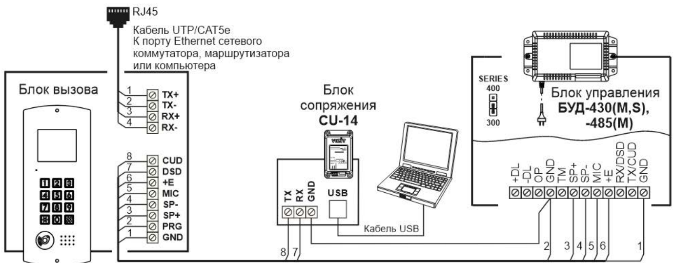
Рисунок 16.1 - Схема соединений блока вызова с блоками управления БУД-430(S, M), -485(M) и блоком сопряжения CU-14
