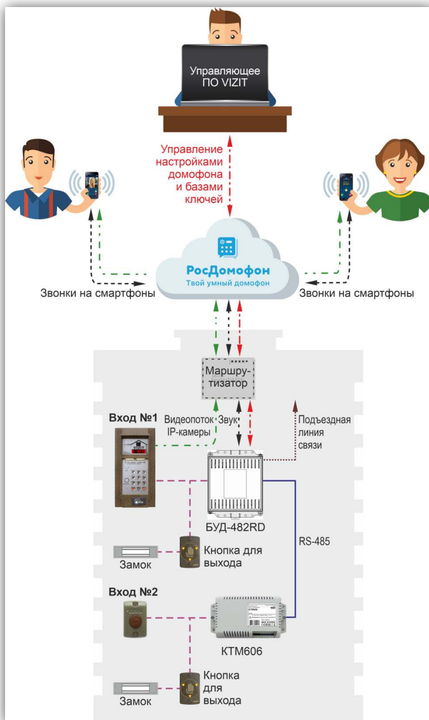
Пример функциональной схемы аналогового + IP-видеодомофона
