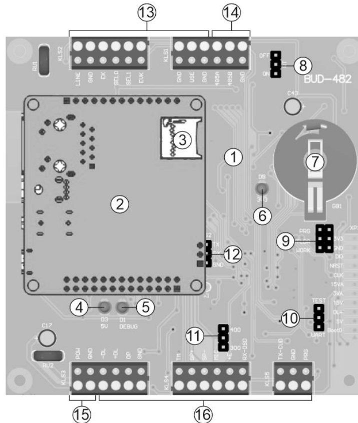
Рисунок 8.1 – Внешний вид плат блока управления
