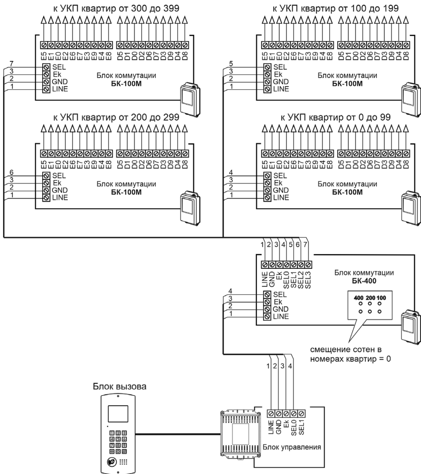
Рисунок 9.11 – Схема соединений блока управления с блоком коммутации БК-400
