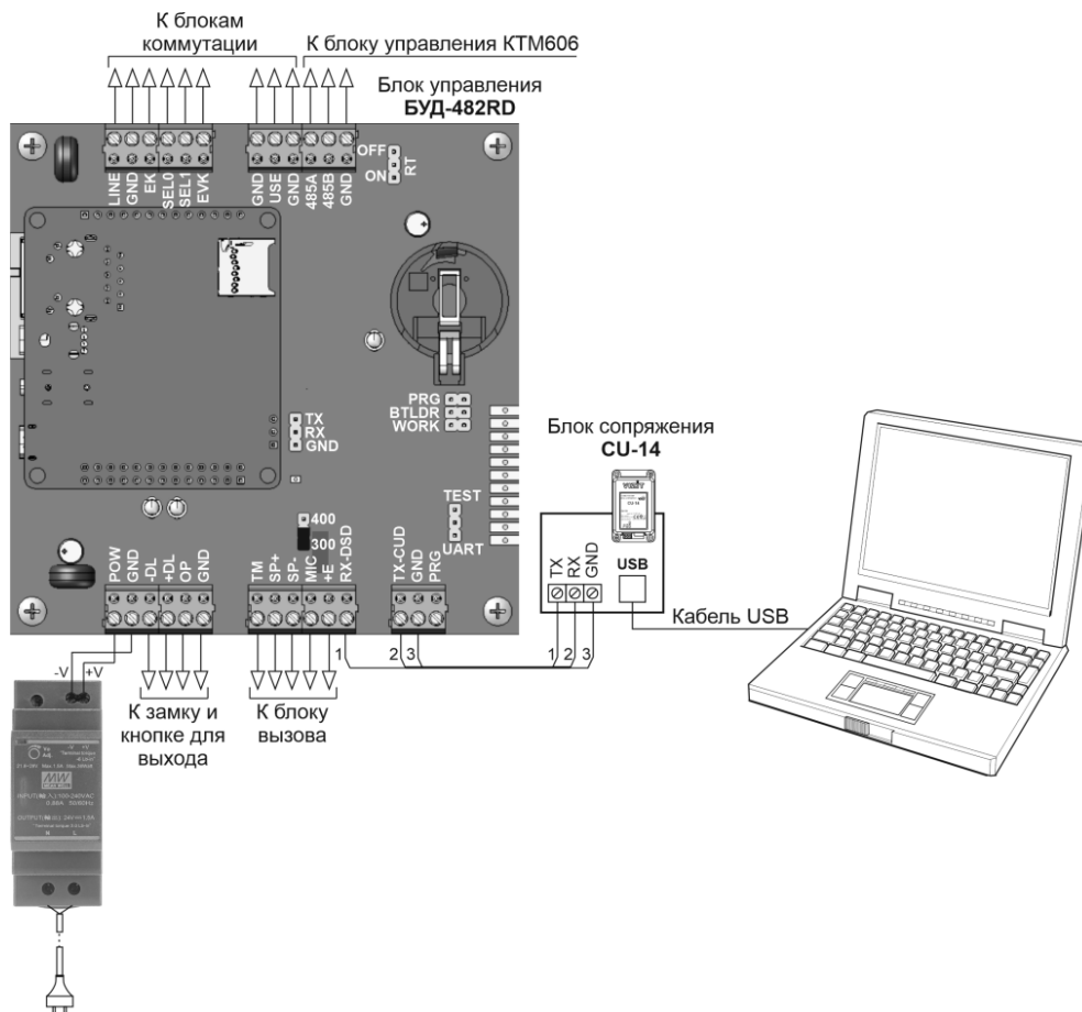
Рисунок 12.1 - Схема соединений блока управления с блоком сопряжения CU-14
