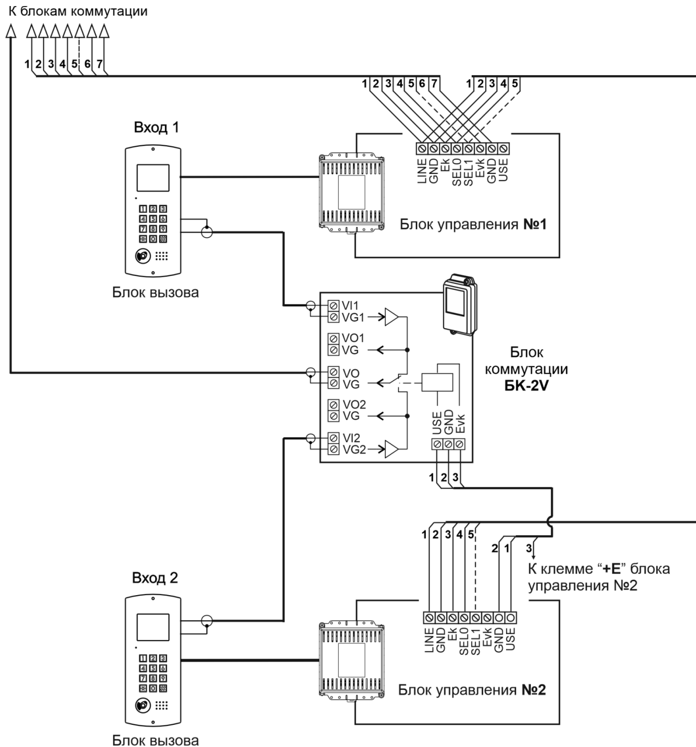
Рисунок 9.11 – Схема соединений блоков управления с блоком коммутации БК-2V
