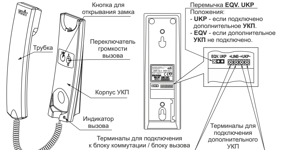
Внешний вид УКП
