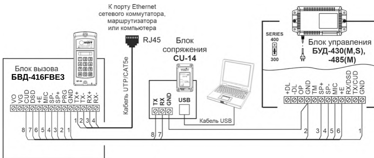
Рисунок 16.1 - Схема соединений блока вызова с блоками управления БУД-430(С, М), -480(С), -485(М) и блоком сопряжения CU-14
