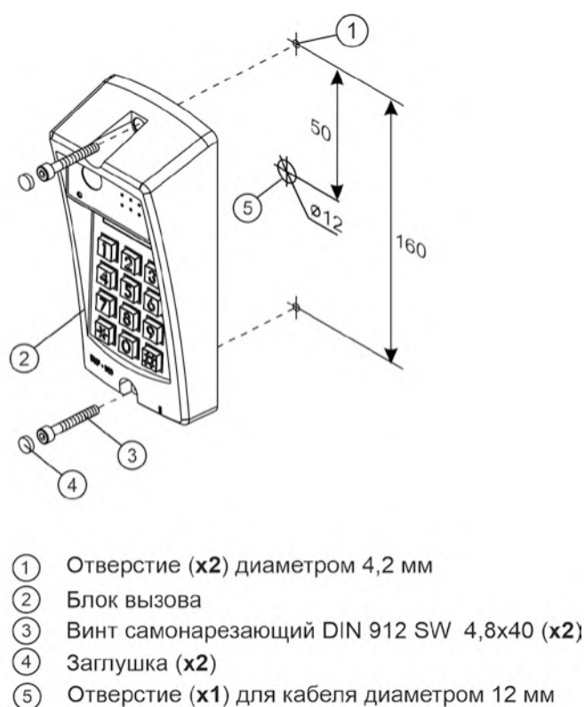
Рисунок 6.3 – Установка блока вызова на неподвижную часть металлической двери
