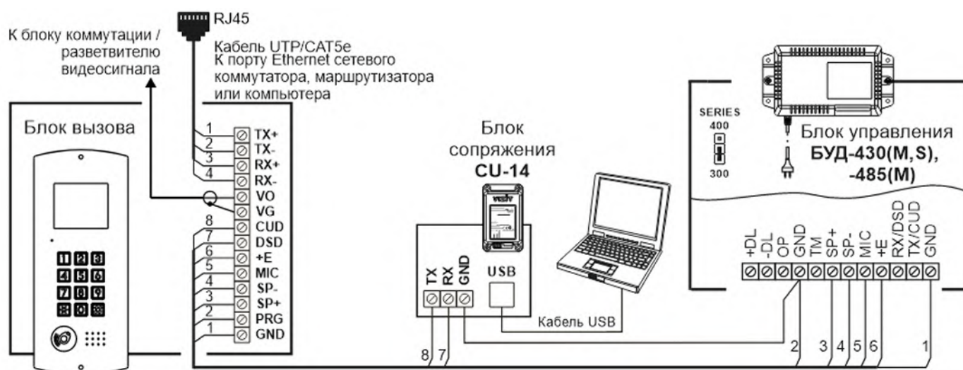
Рисунок 16.1 - Схема соединений блока вызова с блоками управления БУД-430(С, М), -480(С), -485(М) и блоком сопряжения CU-14
