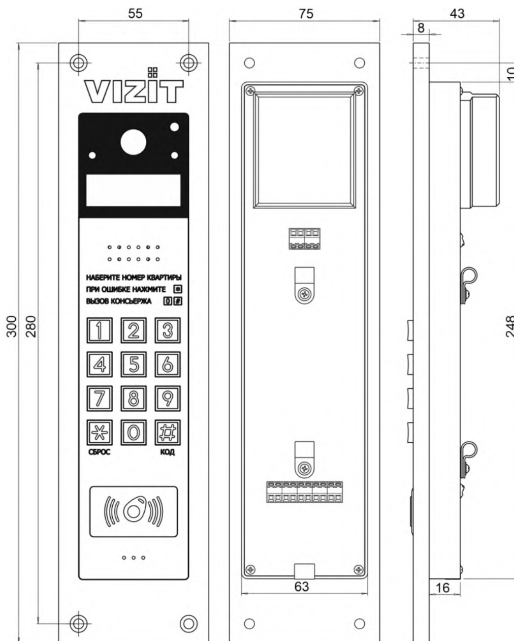
Рисунок 6.2 – Установочные размеры блока вызова
