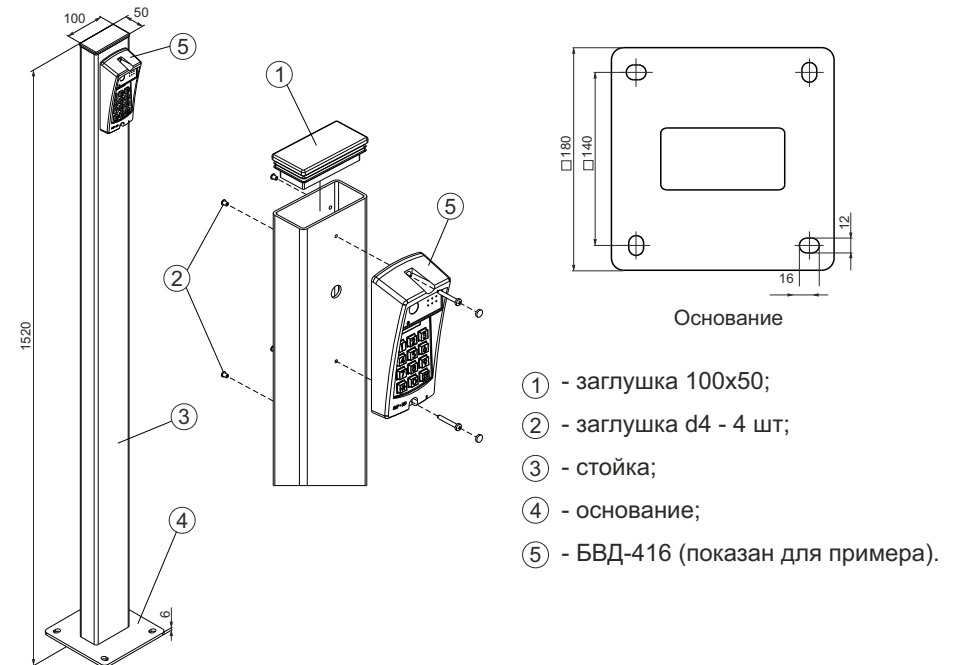
Рис.1 Внешний вид, габаритные и установочные размеры стойки ST10-1
