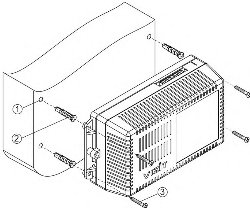
Рисунок 7.2 - Крепление блока управления на стену
