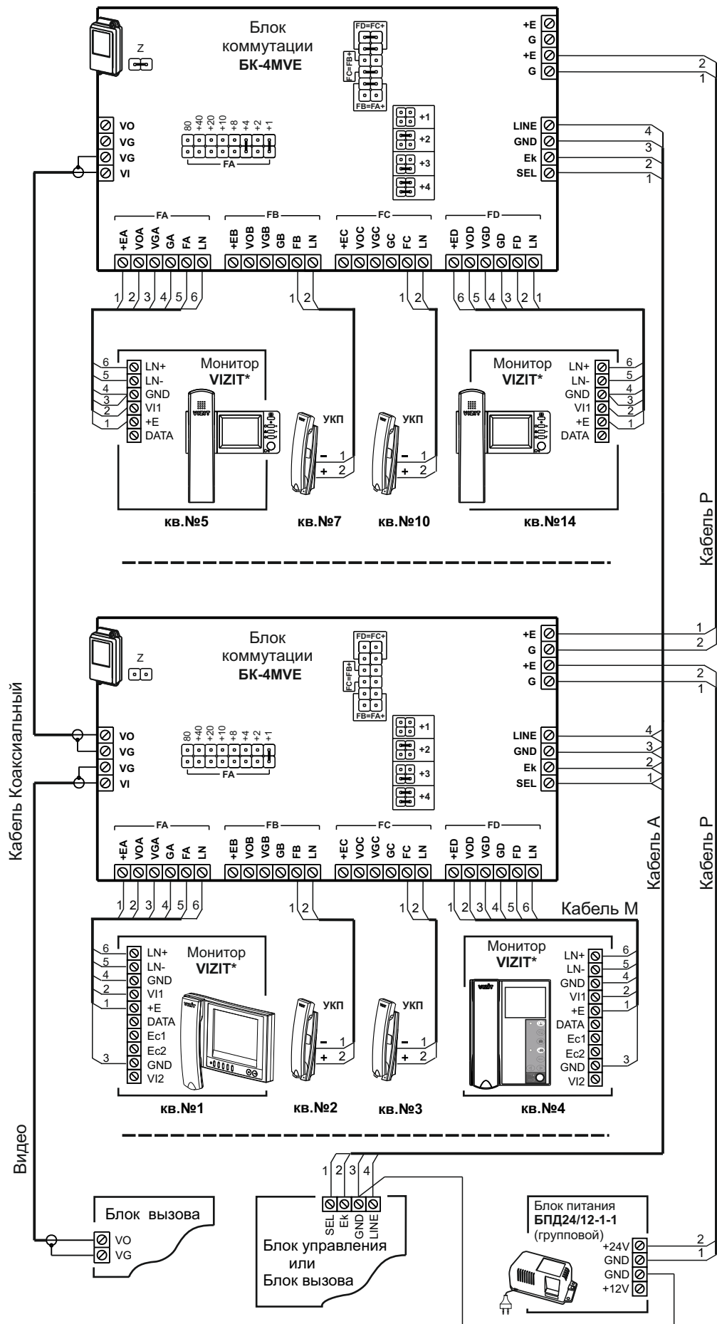
Рисунок 6 - Пример схемы соединений видеодомофона с питанием всех мониторов от группового блока питания
