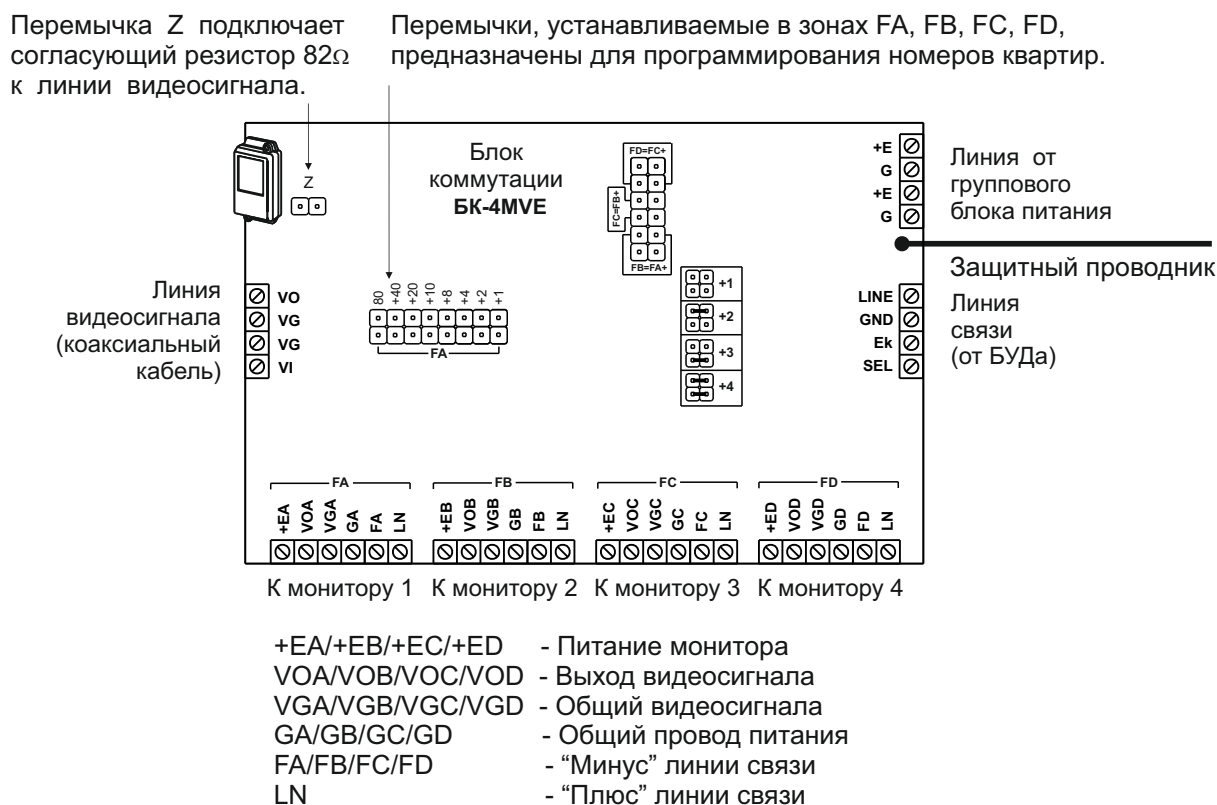
Рисунок 3 - Расположение клемм, назначение цепей и перемычек
